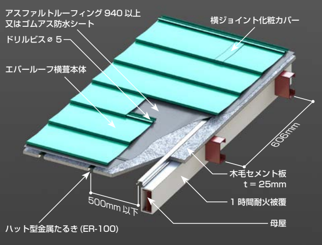
屋根 30分耐火構造
